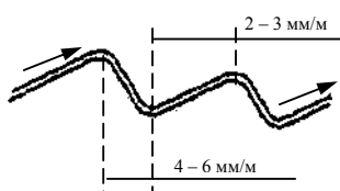
Рисунок 5.6 Трубопровод с переменным уклоном.
