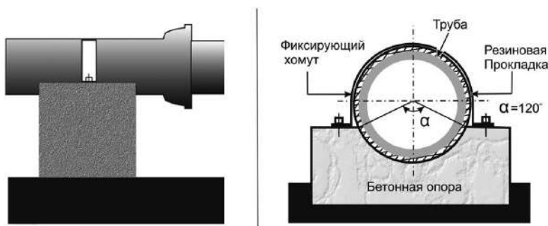
Рисунок 6.14 Крепление трубопровода к опорам.
