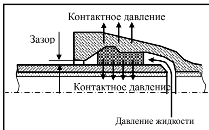
Рисунок 2.16 Контактное давление.
