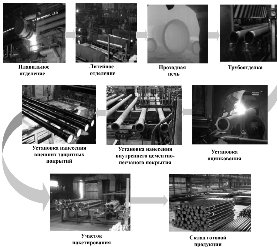
Рисунок 1.2 Технология изготовления труб из ВЧШГ.
