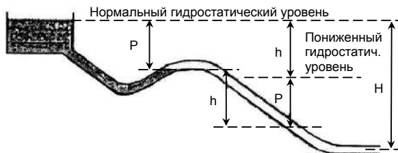
Рисунок 5.3 Условия в гравитационном трубопроводе.
