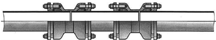
Рисунок 7.7 Ремонт трубопровода при помощи двойного раструба компенсационного ДРК.
