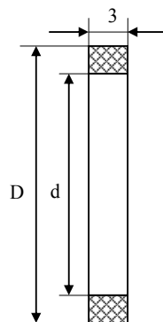
Рисунок 2.15 Уплотнительное кольцо для фланцевого соединения.
