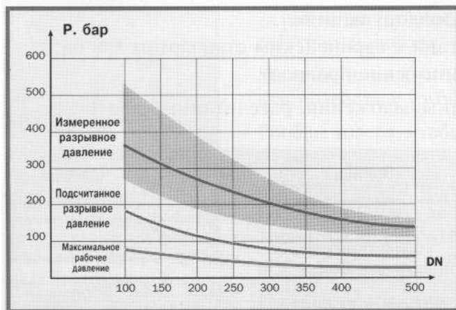
Рисунок 5.1 Трубы ВЧШГ. Давление.
