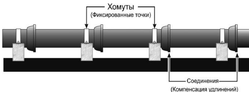
Рисунок 6.15 Компенсация расширений.
