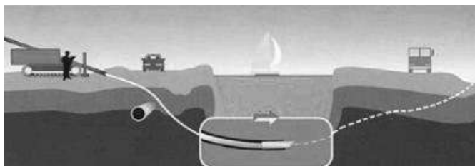
Рисунок 6.18 Бурение пилотной скважины.
