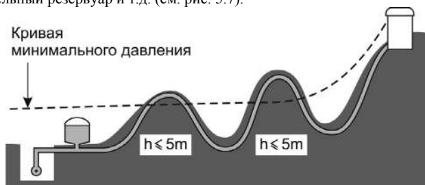
Рисунок 5.7 Трубопровод с уравнильным резервуаром.
