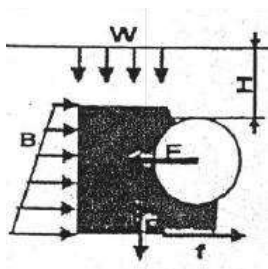
Рисунок 5.9 Активные силы (осевое давление – блок).
