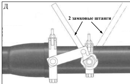
Рисунок 6.7 Типы приспособлений для монтажа и демонтажа труб.
