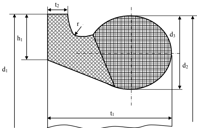
Рисунок 2.3 Уплотнительное резиновое кольцо типа «TYTON».
