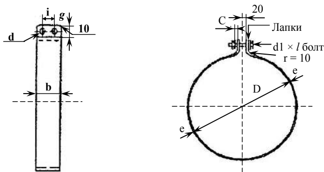
Рисунок 6.8 Медное направляющее кольцо.
