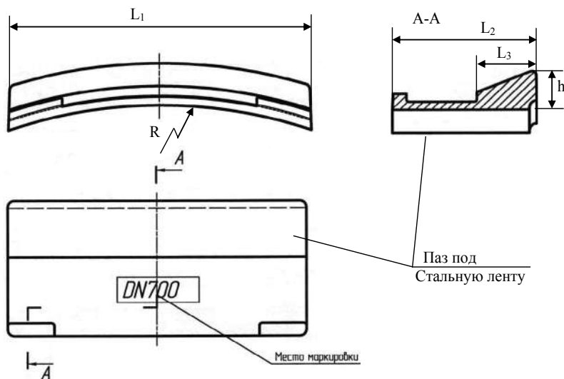
Рисунок 2.11 Стопорные элементы для соединения «RJS».
