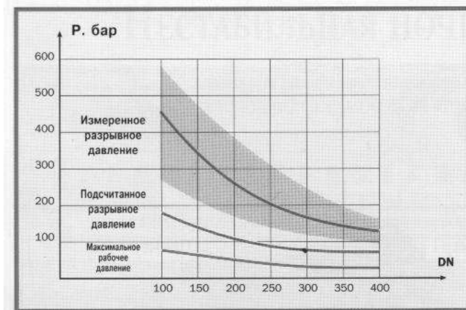
Рисунок 5.2 Фасонные части из ВЧШГ. Давление.
