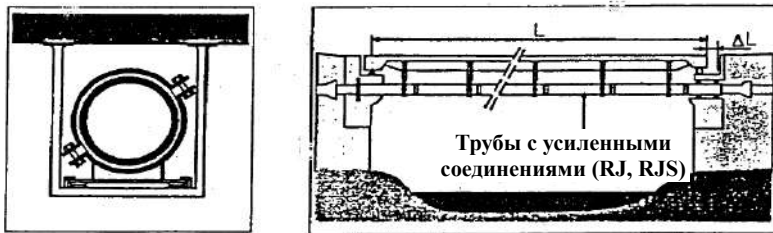
Рисунок 6.31 Трубопровод, закрепленный независимо от сооружения.
