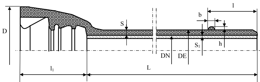
Рисунок 2.6 Труба раструбная с соединением «RJ».
