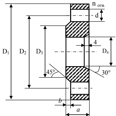
Рисунок 2.14 Фланец из высокопрочного чугуна.
