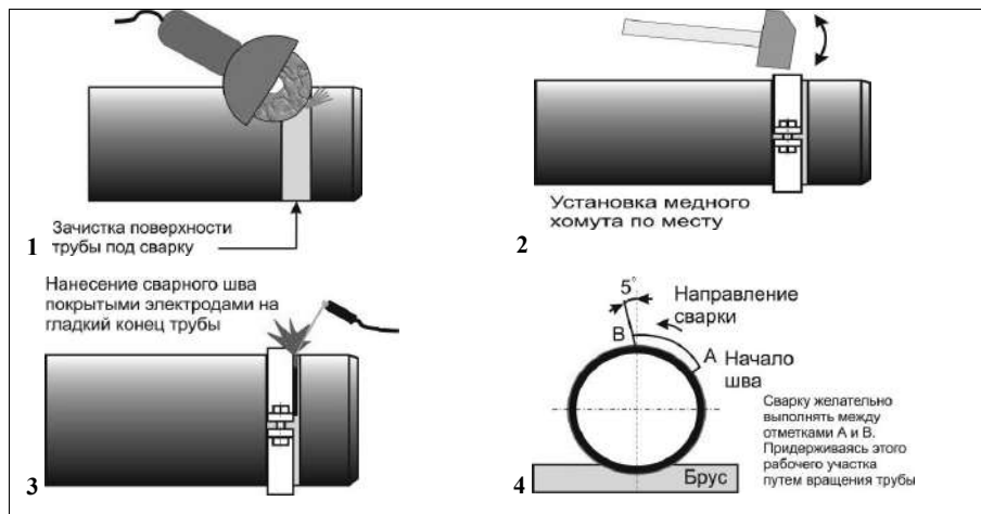
Рисунок 6.9 Технология нанесения наплавленного валика.
