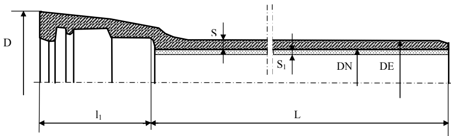
Рисунок 2.2 Труба раструбная с соединением «TYTON».
