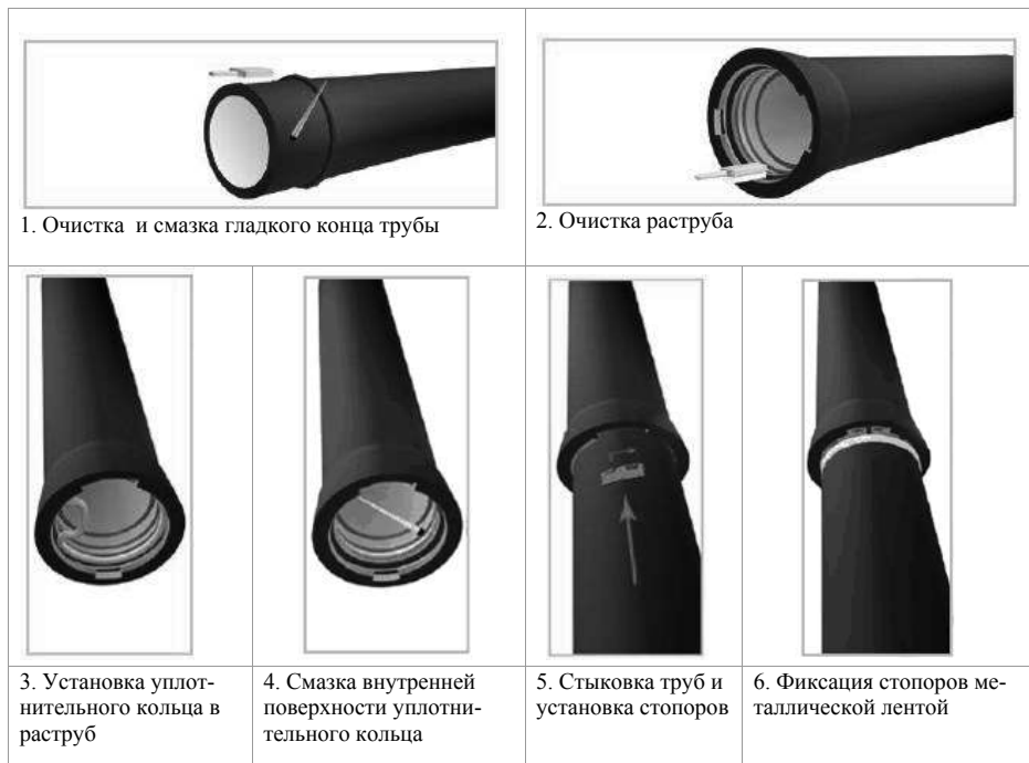
Рисунок 6.6 Монтаж труб с соединением RJS.
