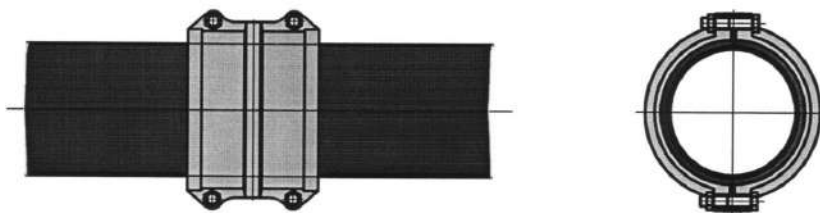
Рисунок 7.8 Ремонт трубопровода при помощи муфты свёртной МС.
