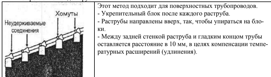
Рисунок 6.30 Способы укладки труб на склонах.
