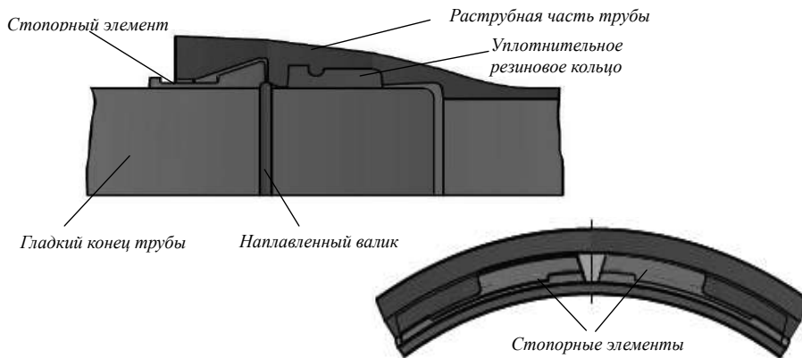
Рисунок 2.9 Раструбно-замковое соединение «RJS».
