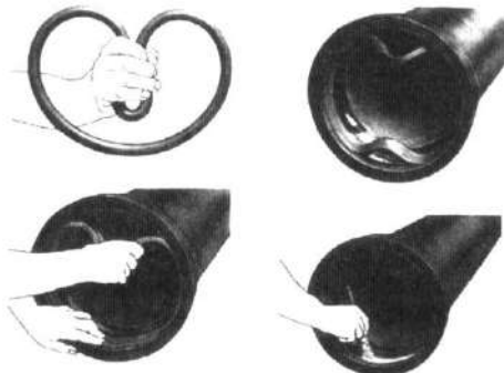
Схема укладки уплотнительного кольца.
