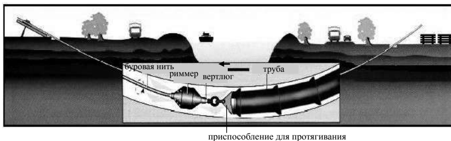
Рисунок 6.20 Протягивание трубопровода.
