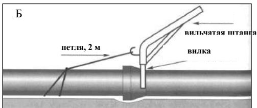
б) при помощи петли и вилочатой штанги
