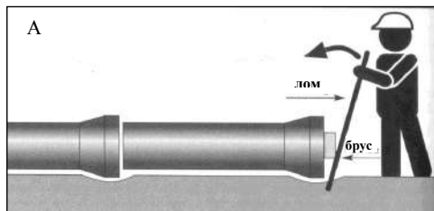
а) при помощи лома и деревянного бруса
