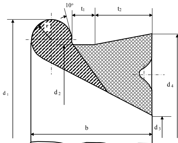
Рисунок 2.7 Уплотнительное резиновое кольцо типа «BPC».
