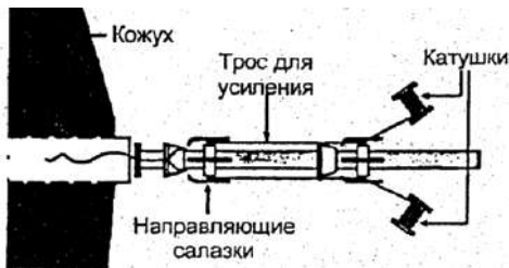
Рисунок 6.33 Укладка трубопровода в кожух.
