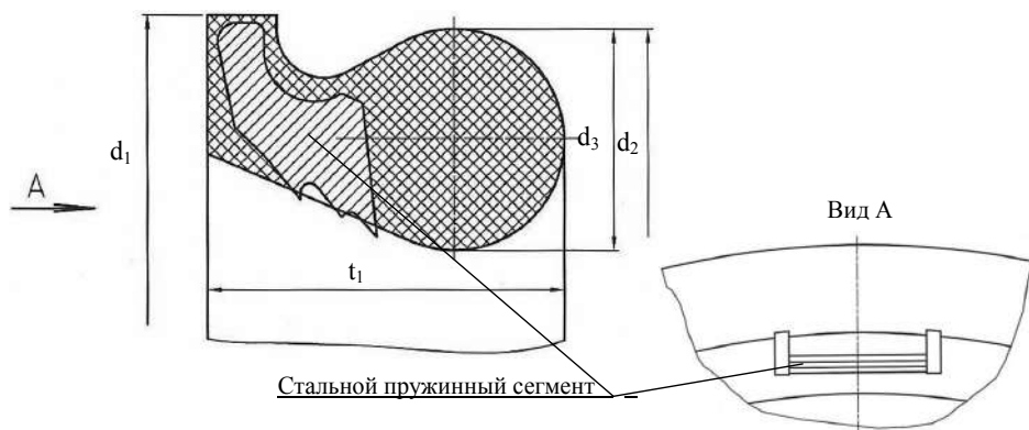
Рисунок 2.4 Уплотнительное резиновое кольцо «TYTON-SIT».
