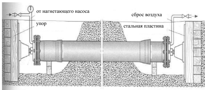
Рисунок 6.34 Гидравлические испытания трубопровода.
