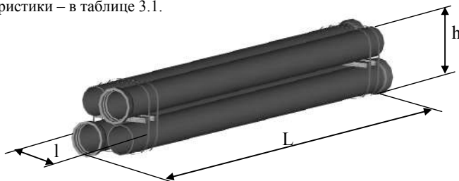
Рисунок 3.1 Пакет труб.
