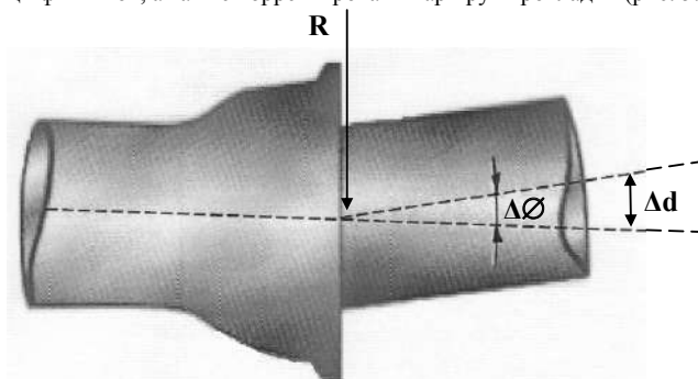
Рисунок 5.10 Допустимый изгиб при укладке.
