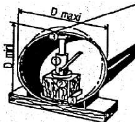
Рисунок 7.5 Восстановление окружности при помощи домкрата.
