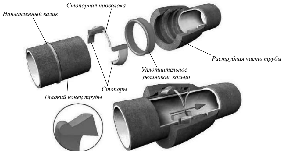
Рисунок 2.5 Раструбно-замковое соединение «RJ».
