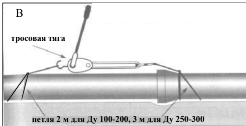
в) при помощи петли и тросовой тяги
