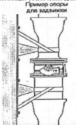
Рисунок 6.29 Укрепление запорной арматуры трубопровода.
