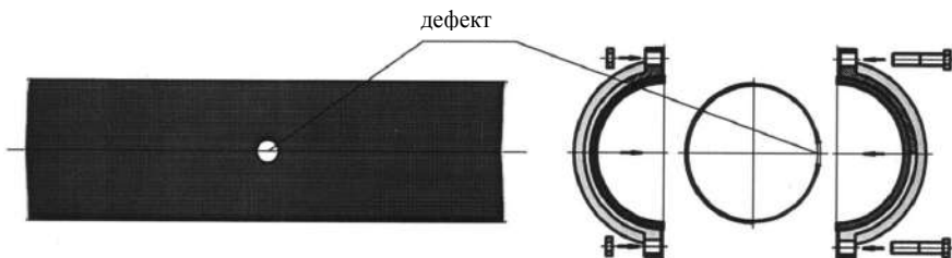
Рисунок 7.7 Ремонт трубопровода при помощи двойного раструба компенсационного ДРК.
