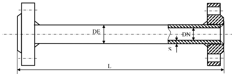
Рисунок 2.13 Труба с приварными фланцами.
